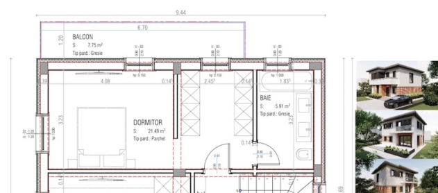
PLAN ETAJ 1
