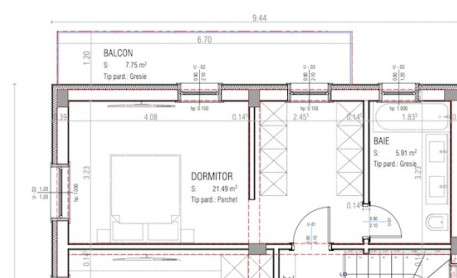
PLAN ETAJ 1
