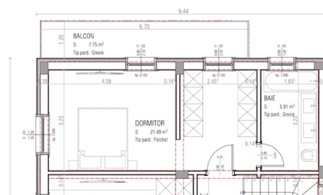
PLAN ETAJ 1
